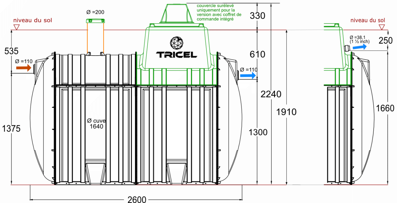
Tricel Novo 6 EH avec écoulement gravitaire (naturel)
